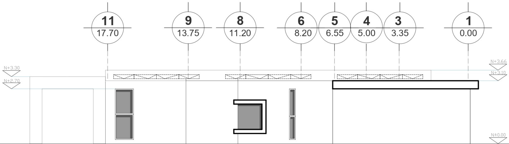
FACHADA NORTE
