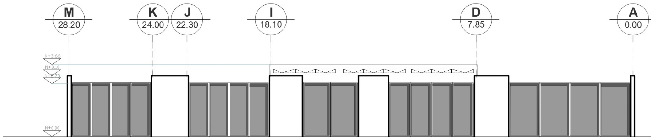
FACHADA OESTE /POSTERIOR
