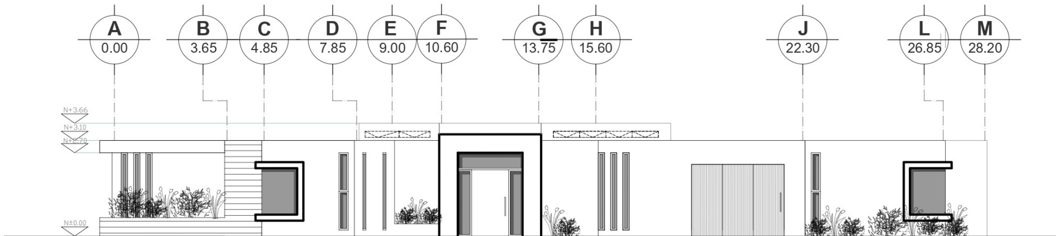
FACHADA ESTE /PRINCIPAL
