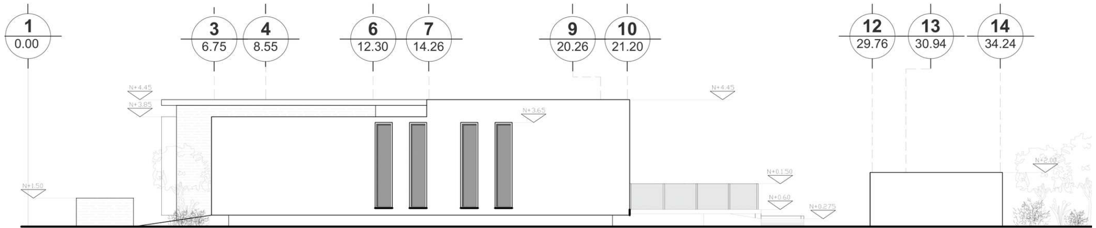
FACHADA NORTE
