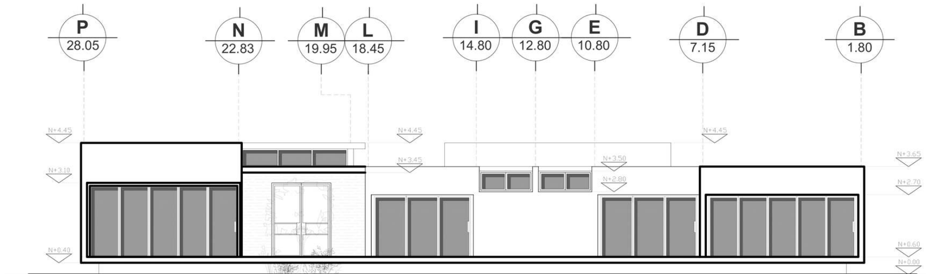
FACHADA OESTE / POSTERIOR
